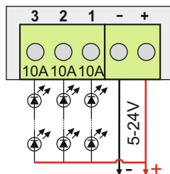
Рис.1 Многопроводная схема
