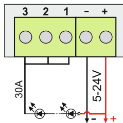
Рис.2 Однопроводная схема
